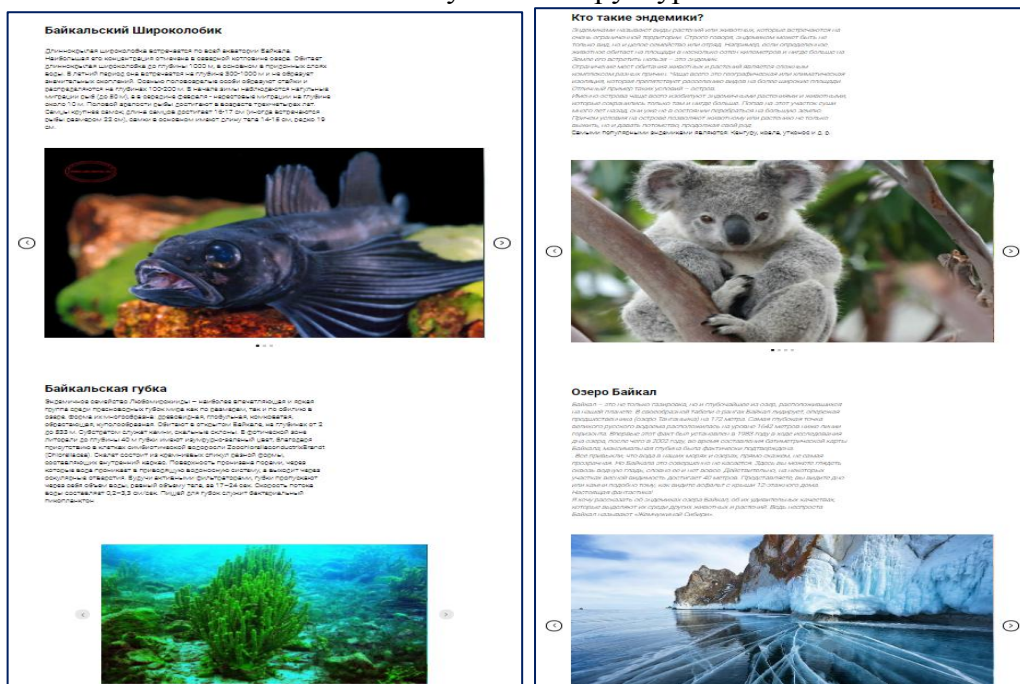
Рисунок 1 – структура сайта
